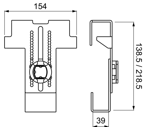
MG-ECU48
