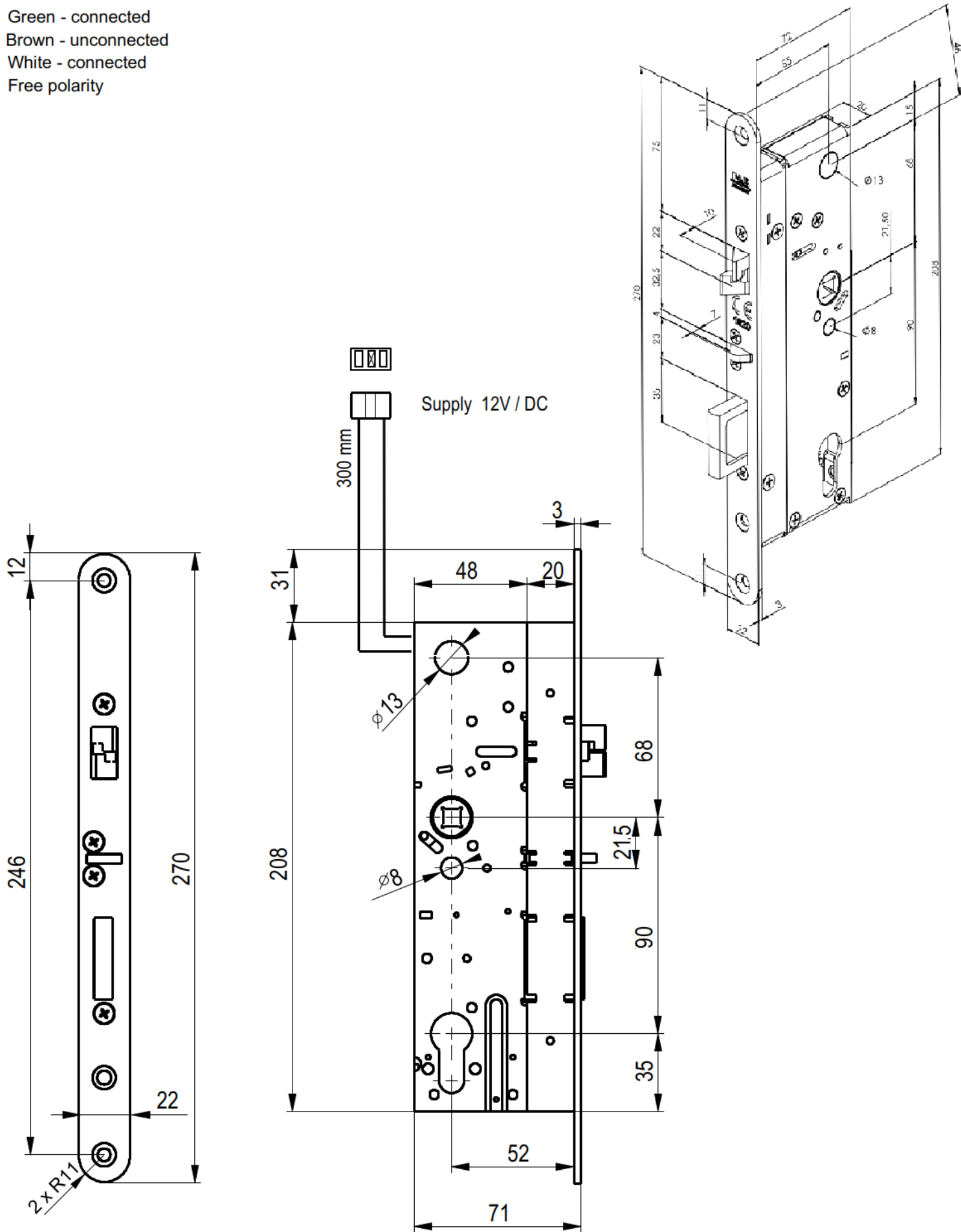
BERA TYPE - E,V Wiring
